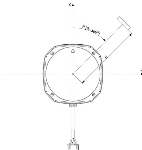
图表 2-4 RPLIDAR S2 扫描数据坐标系定义
