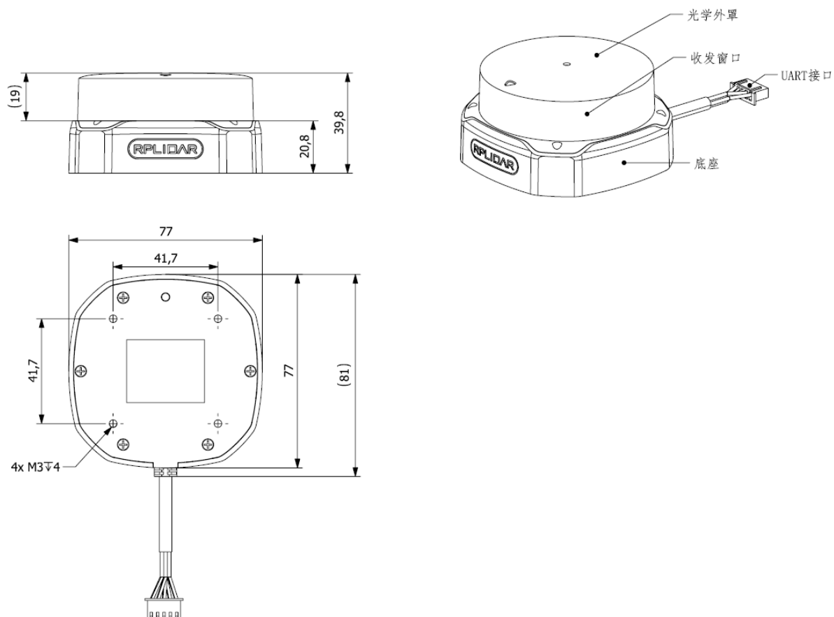
图表 4-1 RPLIDAR S2 机械尺寸图
