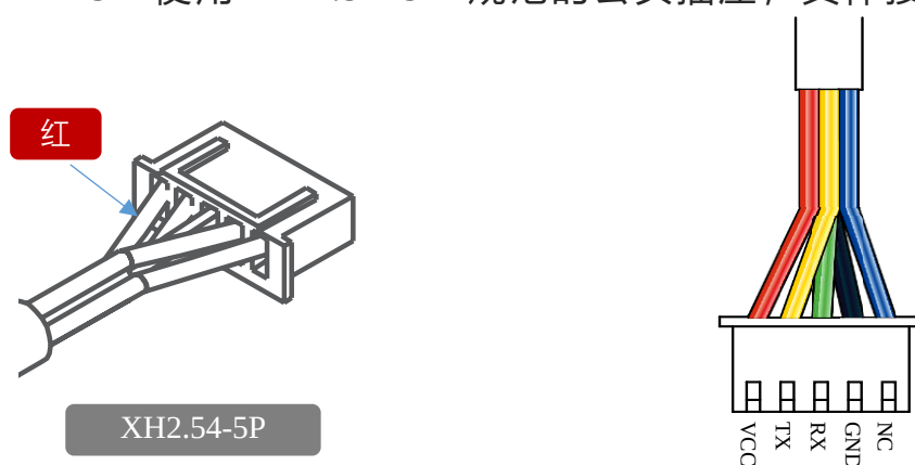
图表 2-5 RPLIDAR 电源接口定义示意图
